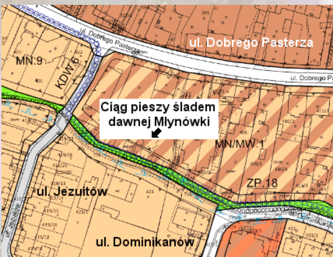
Powyższy rysunek przedstawia fragment projektu planu Prądnik Czerwony – Zachód sankcjonujący brak możliwości przejazdu pomiędzy ul. Lublańską a ul. Dobrego Pasterza wewnątrzsiedlowymi drogami lokalnymi: ul. Dominikanów, Rezedową, Combrową, Jasnorzewskiej. Rozwiązanie to zostało wprowadzone na wniosek mieszkańców i wynikało z analizy modelu ruchu samochodowego w tym rejonie. Zamiast połączenia drogowego ul. Dominikanów i Jezuitów, został wprowadzony ciąg spacerowy śladem dawnej Młynówki.
